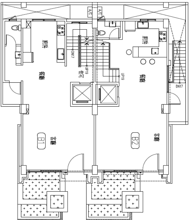
壹層平面圖 SCALE:1/100
