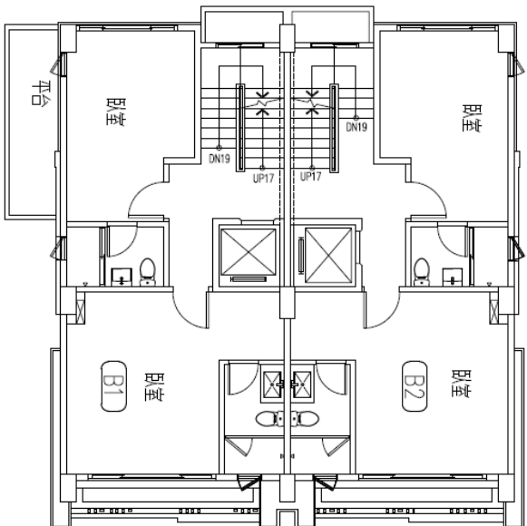
貳層平面圖 SCALE:1/100
